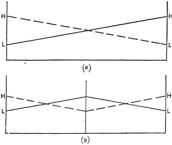
चित्र ८६—(a) एकनिष्पंदीय और (b) द्विनिष्पंदीय दोलन प्रणालियाँ।
